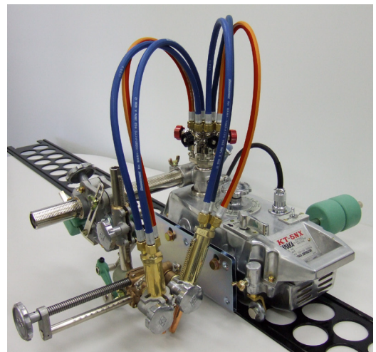
必要部品を追加いただくことでY開先、X開先切断も可能です。 (写真はY開先仕様)
